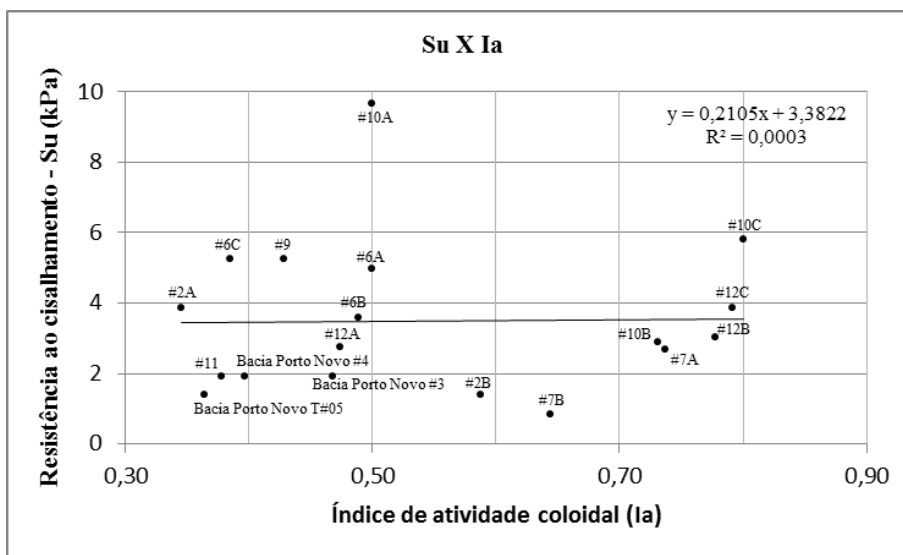
Figura 11. Resistência ao cisalhamento versus % Ia.
