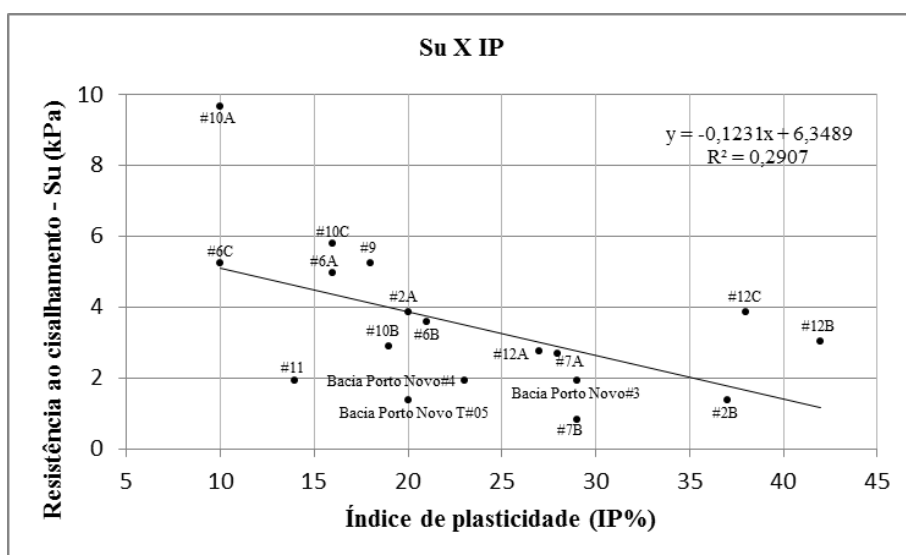
Figura 10 - Resistência ao cisalhamento versus IP.
