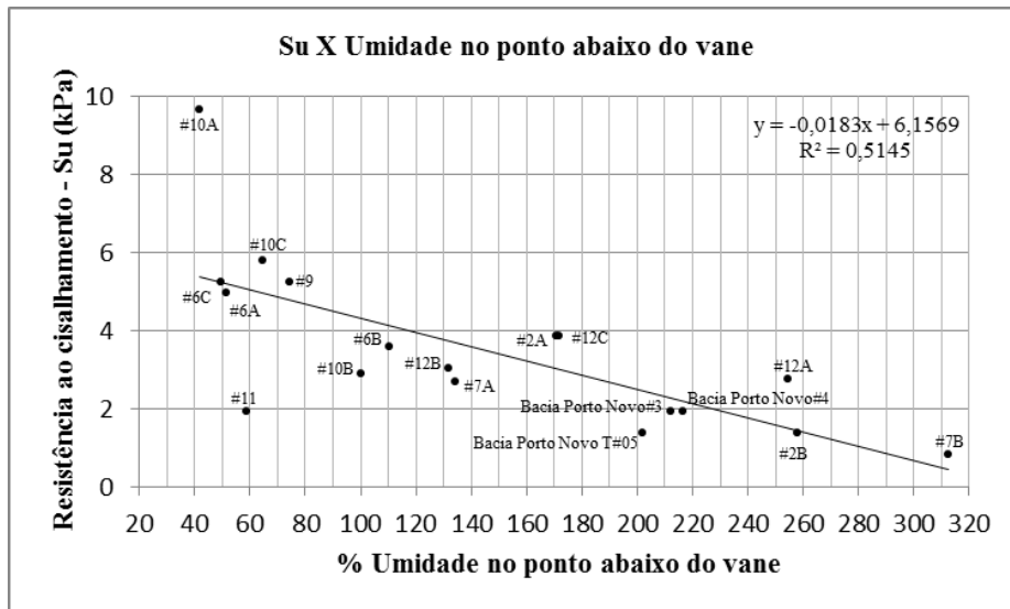
Figura 8 - Resistência ao cisalhamento versus Umidade no ponto abaixo do vane.
