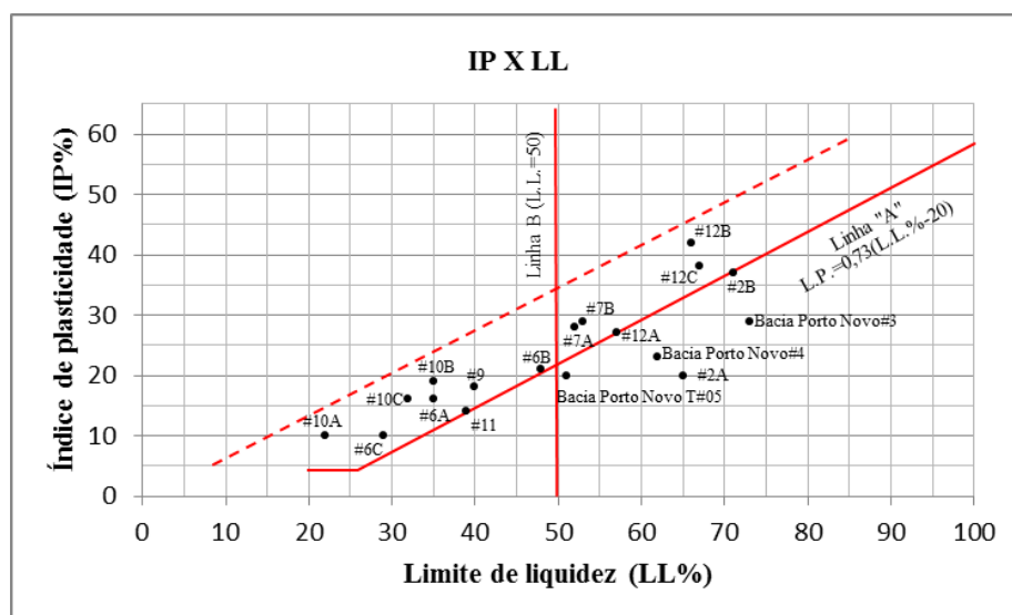
Figura 6 - Carta de plasticidade de Casagrande.
