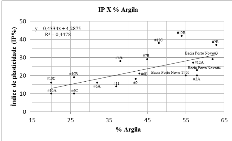
Figura 7 - Índice de plasticidade versus % Argila.
