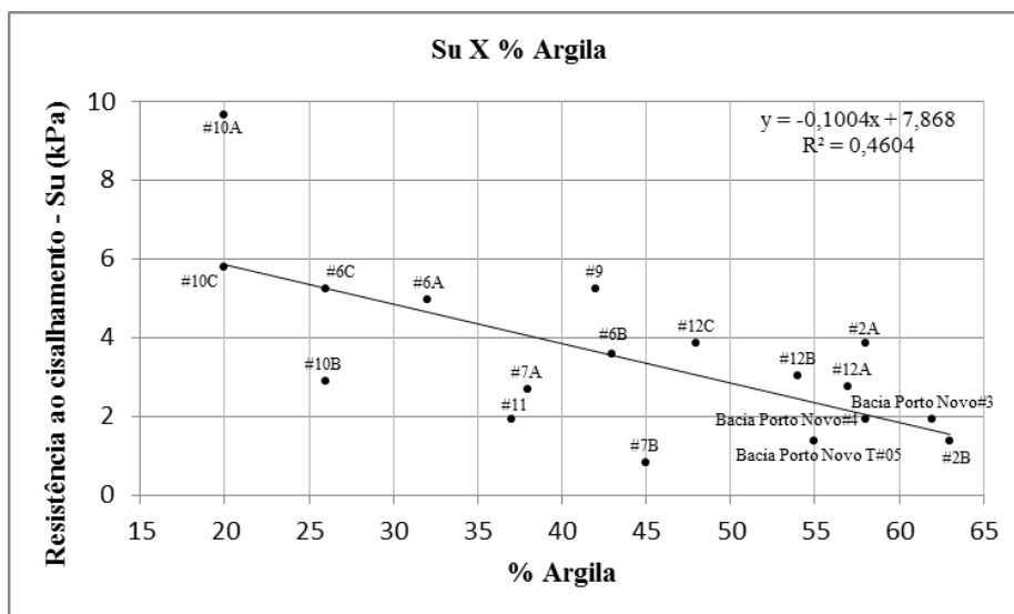
Figura 9 - Resistência ao cisalhamento versus % Argila.
