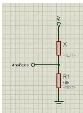
Figura 2 - Circuito para leitura de resistência.
