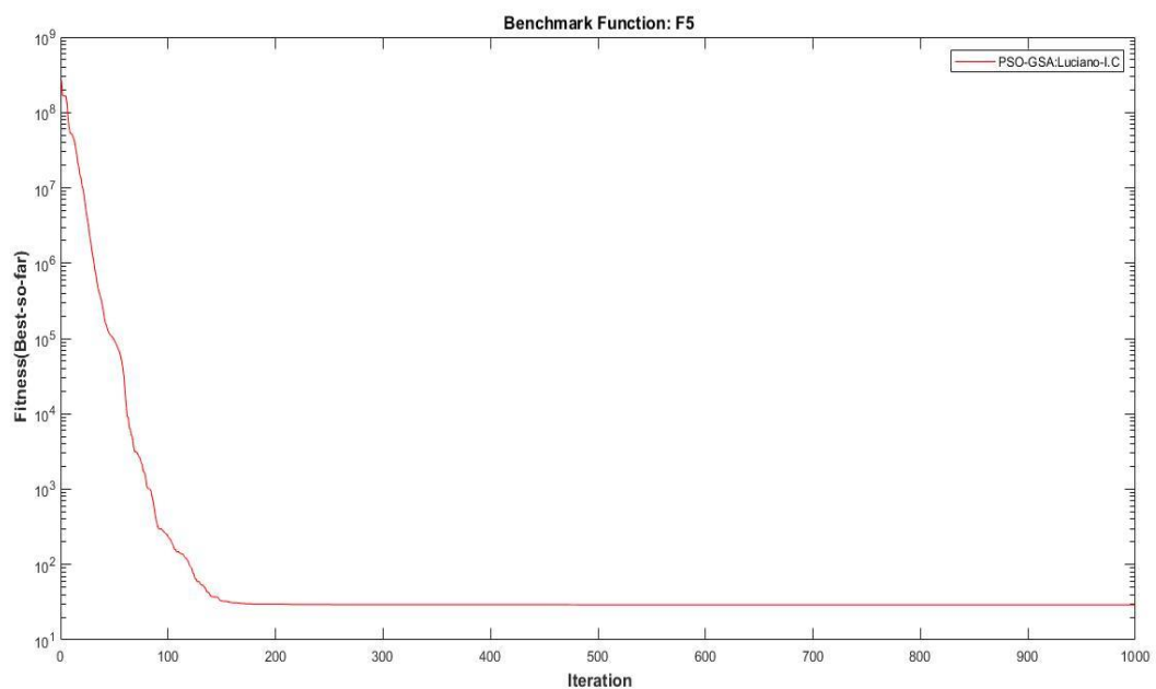
Figura 1. Implementação do PSO-GSA usando a função 5.
