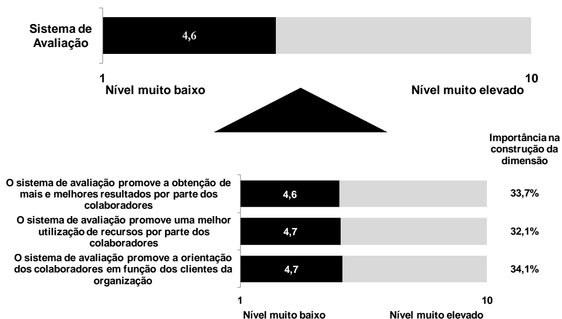
Gráfico 1 – Variável latente sistema de avaliação de desempenho e respetivas variáveis de medida constituintes
