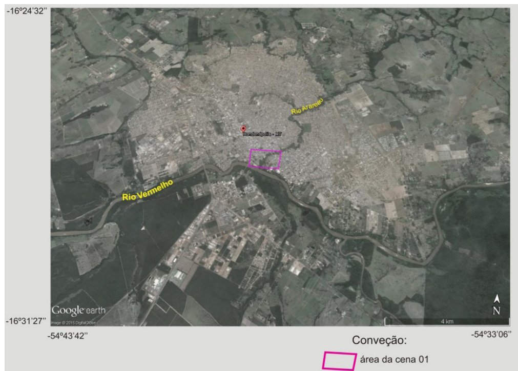
Figura 2 – Áreas de muestreo (cena 01) de los datos de uso y ocupación de la tierra de la zona de preservación del río Arareau en su confluencia con el río Vermelho en Rondonópolis, MT
